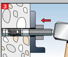
Anker einschlagen durch Setzlehre
