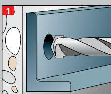
Bohrloch erstellen
