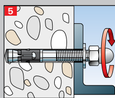
Hutmutter aufdrehen
