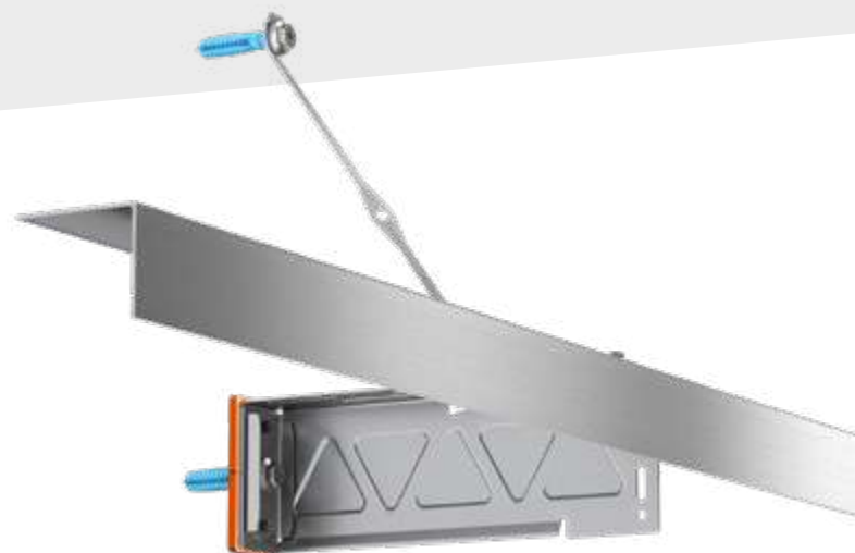
Horizontale Montage
