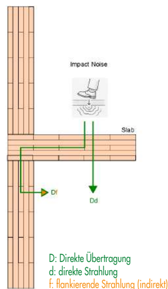
Abbildung 3 Übertragungswege Trittschall
