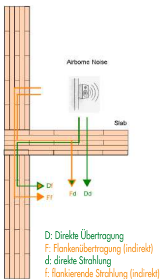
Abbildung 2 Übertragungswege Luftschall
