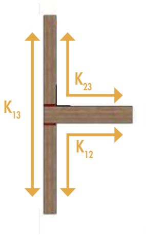
Abbildung 1 Stoßstellendämmmaß Prüfung K_{ij} K_{13} : Wand, K_{23} : Wand-Decke, K_{12} : Decke-Wand
