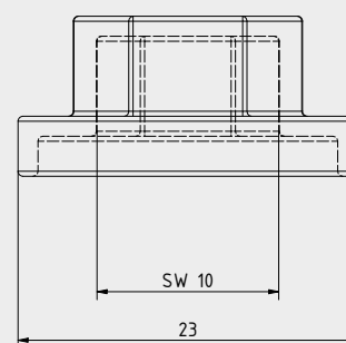
Seitenansicht
