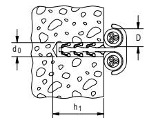
Steckfix plus Zwillingsschelle SF plus ZS
