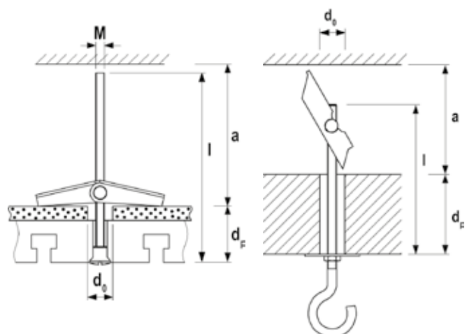
Federklappdübel mit Haken KDH 4
