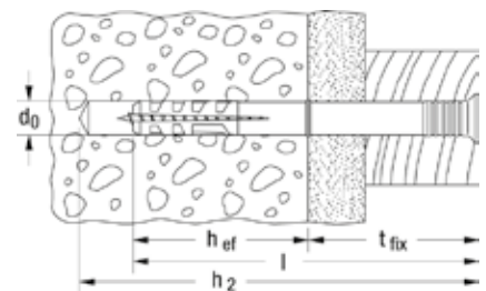
Nageldübel N-S - Senkkopf, vormontiert mit galvanisch verzinkter Nagelschraube
