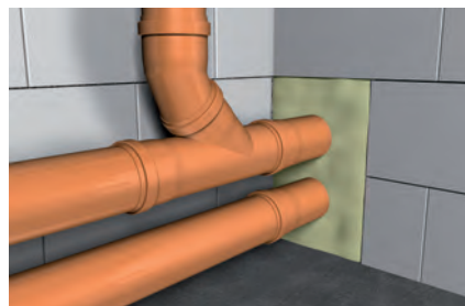
Füllen von Rohrdurchführungen
