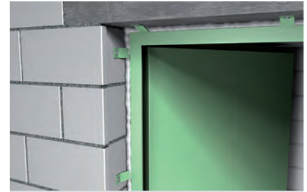
Ausschäumen von Stahltürzargen
