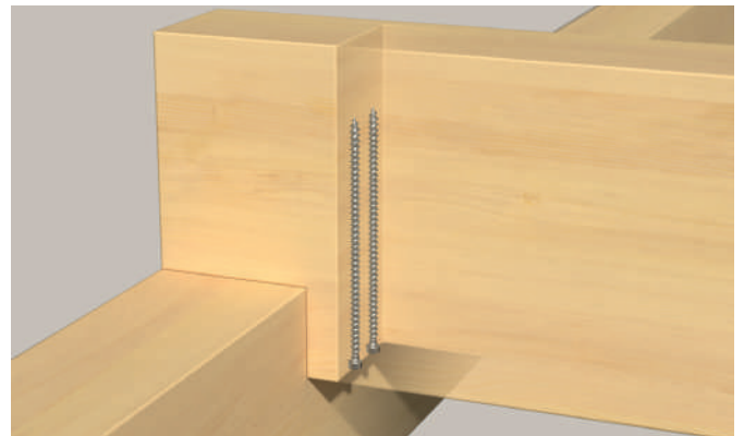
Ausklüftung (Verstärkung am ausgeklüfteten Auflager)
