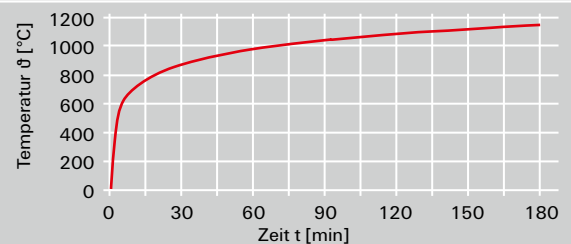
Bild 2: Einheitstemperaturkurve nach DIN EN 1363-1
