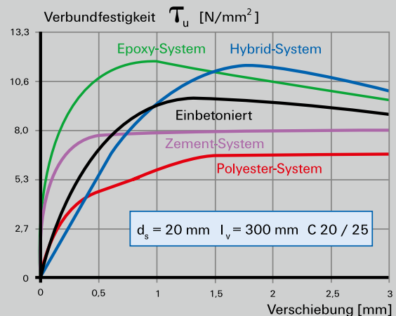
Bild 1: Last-Verschiebungsverhalten einbetonierter und eingemörtelter Stäbe (Quelle: Spieth, H.; Eligehausen, R. (2002): Bewehrungsanschlüsse mit nachträglich eingemörtelten Bewehrungsstäben. Beton- und Stahlbetonbau 97, Heft 9, 2002.)
