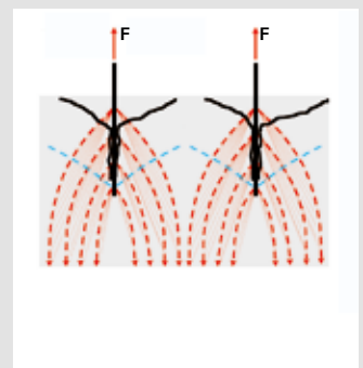
Bild 2: Lastweiterleitung eingemörtelter Stäbe (Spieth, 2002) ohne Anschlussbewehrung
