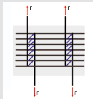
Bild 1: Lastweiterleitung eingemörtelter Stäbe (Spieth, 2002) mit Anschlussbewehrung
