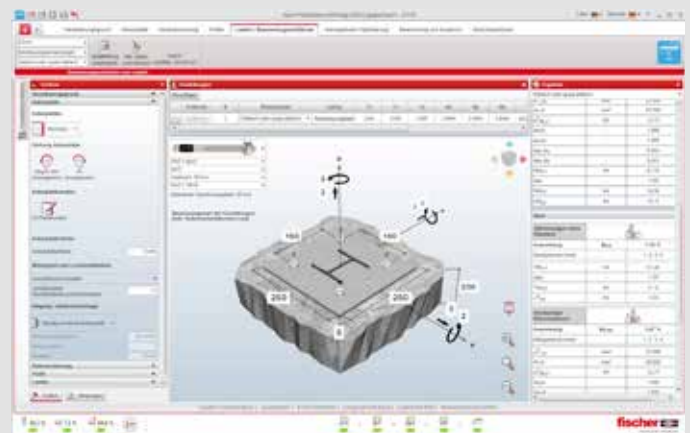
Bild 4: Bemessungssoftware FIXPERIENCE, Programm-Modul C-FIX
