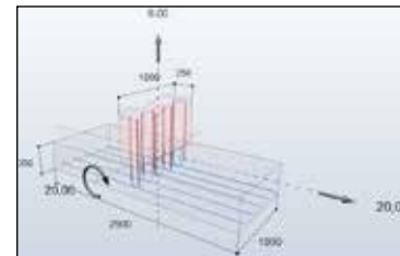
Anschluss Wand/Fundament
