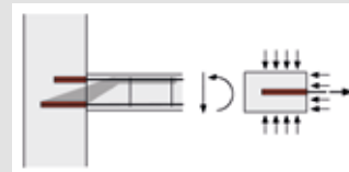
Bild 3: Eingemörtelte Stäbe im Bereich von Endauflagern
