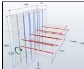
Anschluss Platte/Wand
