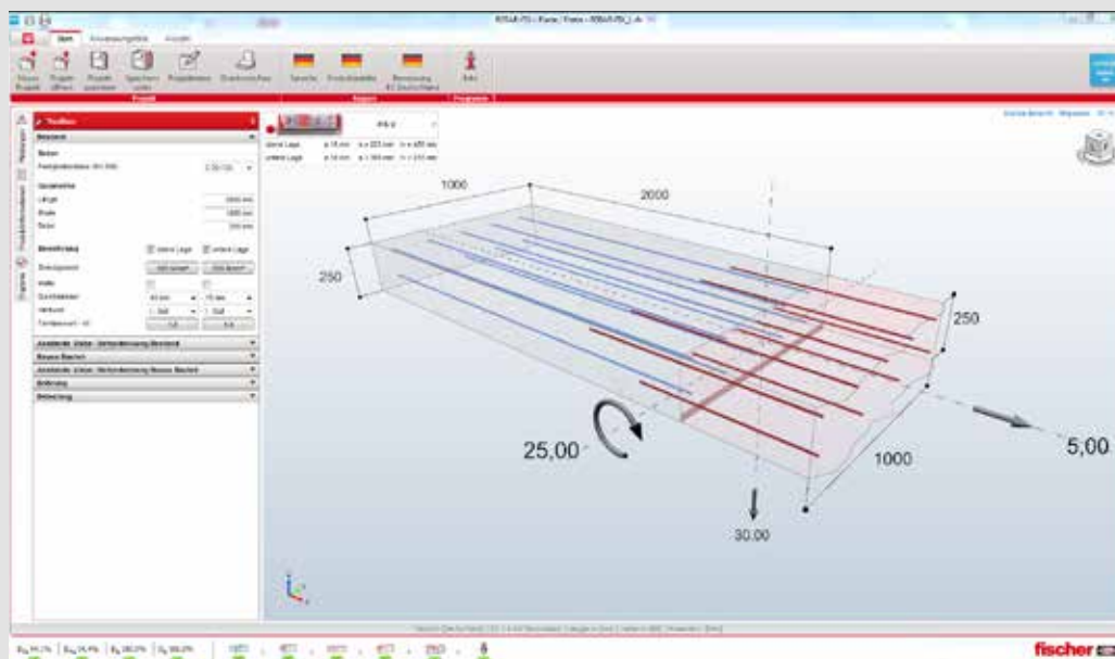
Anschluss Platte/Platte
