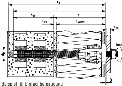
Beispiel für Einfachbefestigung
