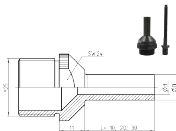
SL-Mundstück FireBird® Pro/FireFox®
