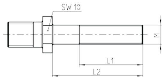
Standard-Gewindedorn FireBird®
