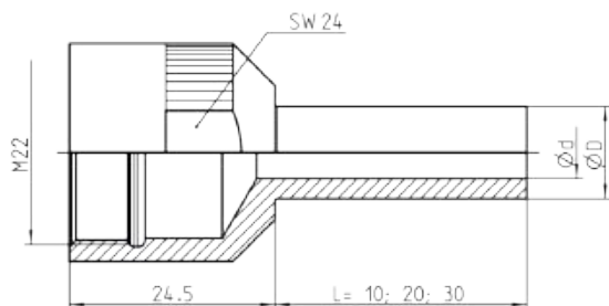
SL-Mundstück FireBird®
