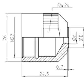
Standard-Mundstück FireBird®
