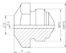
Sonder-Ausführung 17/.....MB-Mundstücke
