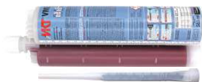
Kartusche VME plus 585 Side-by-side Kartusche Inhalt: 585 ml
