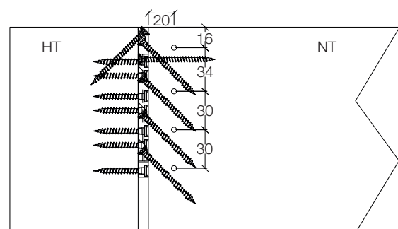
Ansicht Schraubenpositionierung
