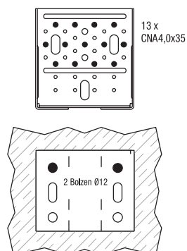
Nagel-/Bolzenbild: A
