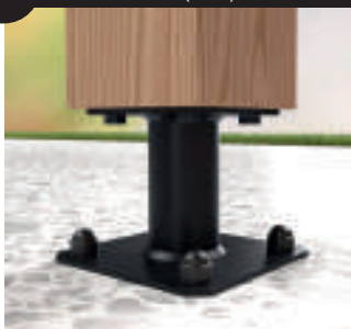
3 Stützenfuß (fest)
