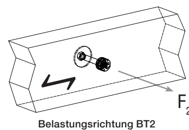
Belastungsrichtung BT2
