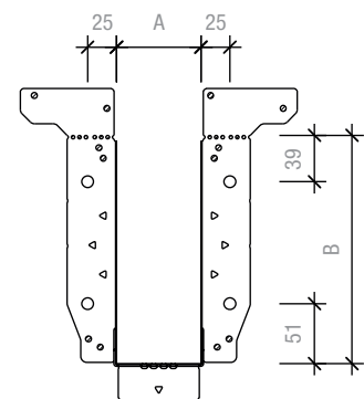
Lage der Bolzenlöcher
