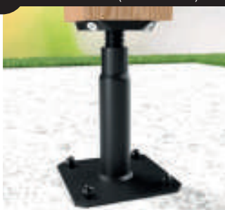
5 Stützenfuß (verstellbar)
