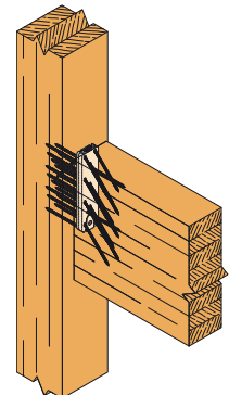
Nebenträger an Stütze
