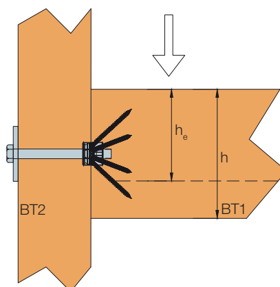
Querzugrelevante Maße im BT1
