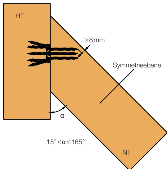
Draufsicht Schräganschluss
