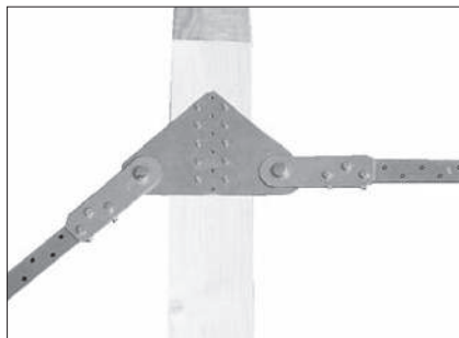
Detail am Firstpunkt:
