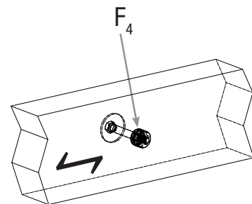
Belastungsrichtung BT2
