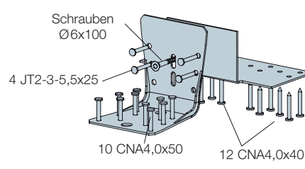
Holz-Holz-Anschluss
